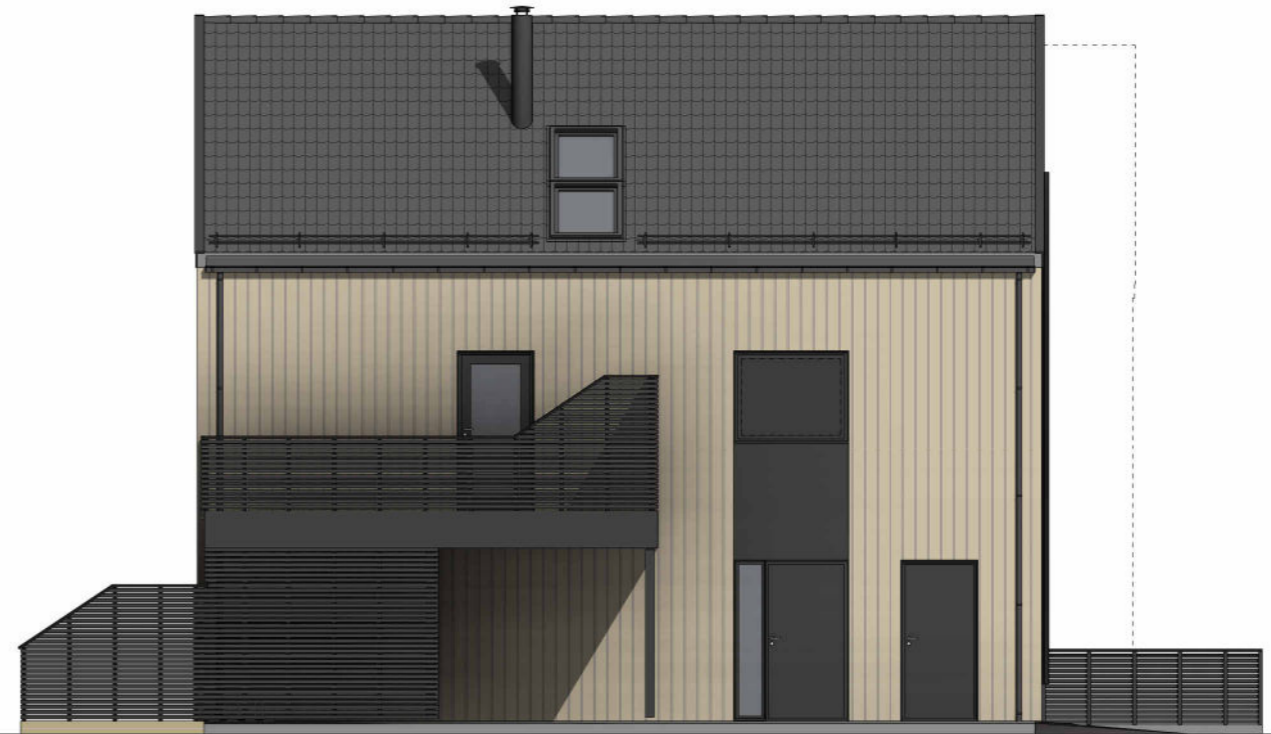
sør-sørvest 1 : 100
